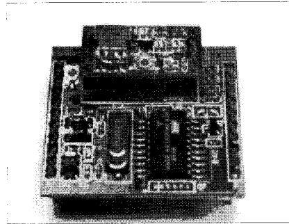
그림 2 무선 송신기 모듈 Fig. 2. Wireless Transmitter Module
