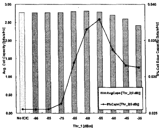
그림 3. Thr_1에 따른 Capacity 성능
