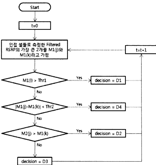
그림 1. Threshol-Based Region Decision 알고리즘 순서도
