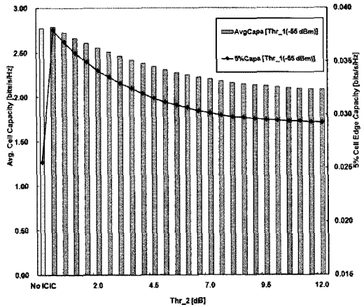
그림 4. Thr_2에 따른 Capacity 성능
