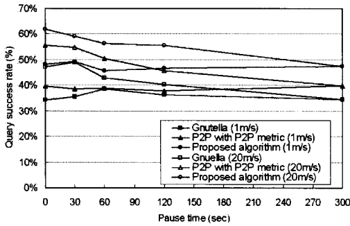
그림 3. 쿼리 성공률
