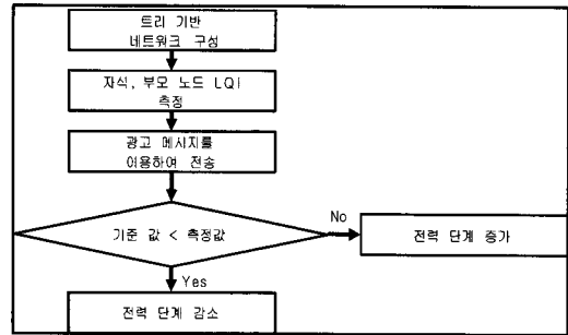
그림 1. 송신전력제어 과정
