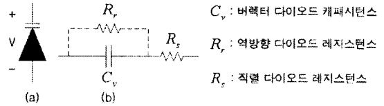
[그림 5] (a) 버렉터 다이오드의 기호; (b) 등가 모델
