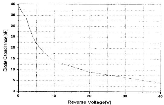
[그림 6] 역전압에 따른 버렉터 다이오드의 캐패시턴스 특성
