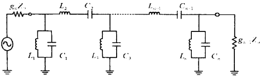
[그림 1] 일반적인 대역통과여파기
