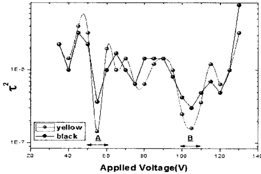
[그림 4] 인가펄스에 의한 대전입자응답속도
