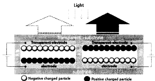
[그림 1] 대전입자형 디스플레이 구동원리
