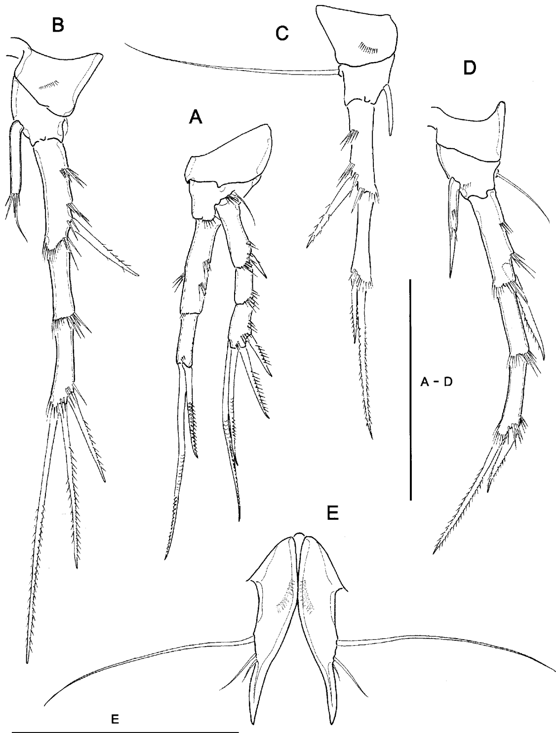
Fig. 3. Parastenocaris ondali , n. sp., female. A-E, legs 1-5. Scale bars: A-E=50 \mu m.
