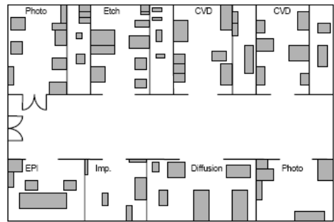
그림 3. 레이아웃
