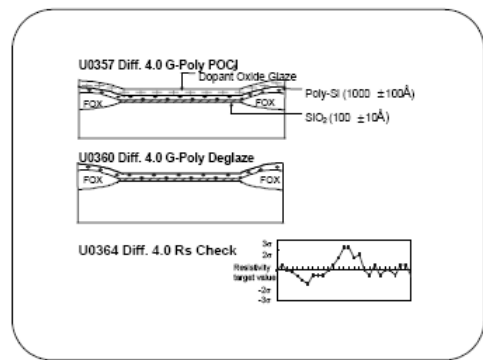
그림 6. 단면도
