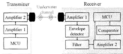
그림 2. 블록다이어그램
