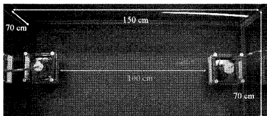
그림 7. 구조 실험 환경
