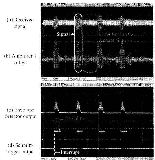
그림 5. 수신부의 신호처리
