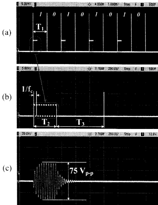
그림 4. 송신부의 신호처리
