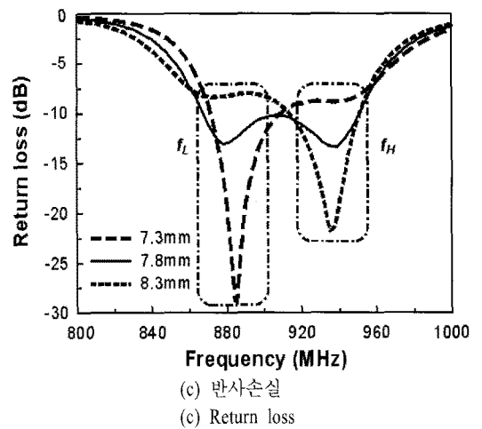
그림 3. 사각 형태의 급전부 좌우 길이( L_4 ) 변화에 따른 특성 변화
