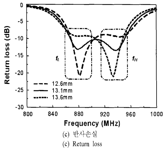
그림 2. 사각 형태의 급전부 상하 길이( L_3 ) 변화에 따른 특성 변화
