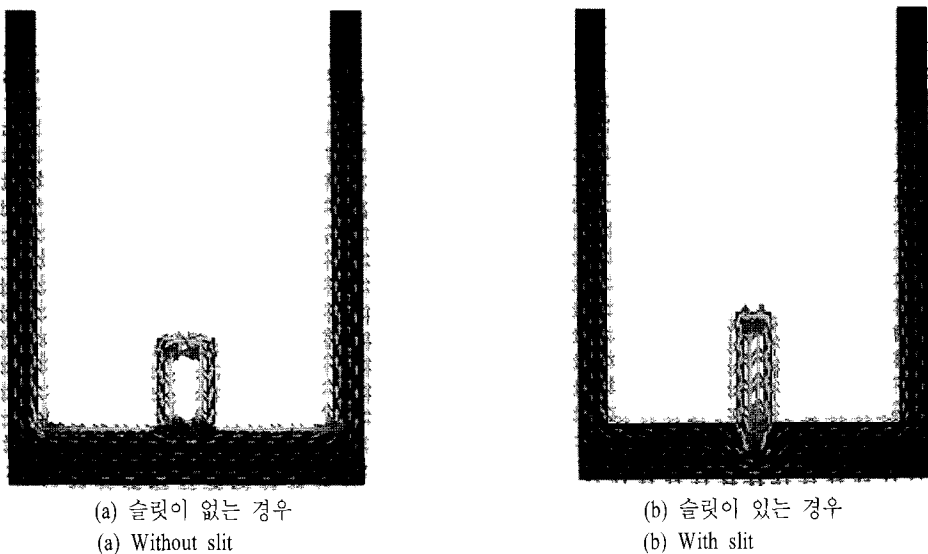
그림 9. 최적화된 태그 안테나의 전류 분포
