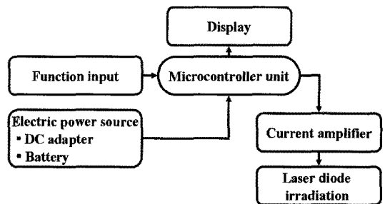
그림 1. 기기의 구성도.
