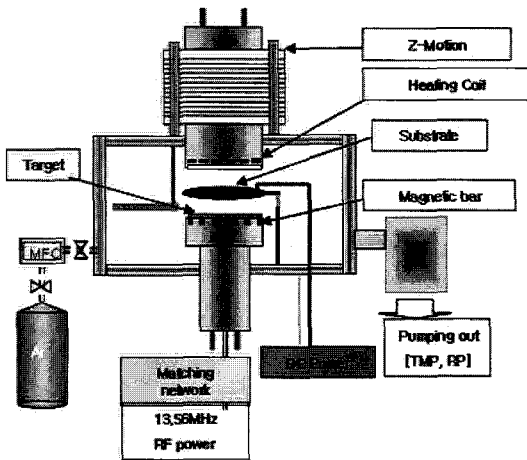
그림 1. RF 마그네트론 스퍼터 장치도.
