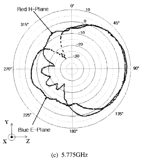
그림 8. 제안한 안테나의 방사패턴 (a) 5.150GHz (b) 5.350GHz (c) 5.775GHz Fig. 8. Radiation pattern of the proposed antenna
