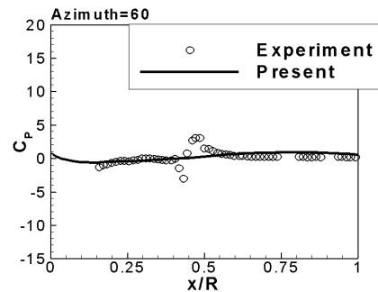
(d) Azimuth=60 deg
