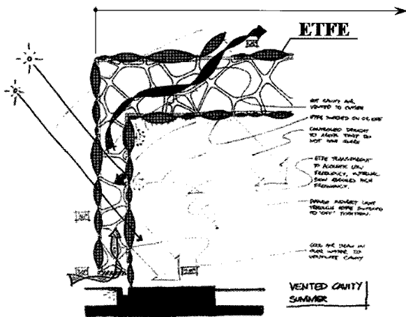
〈그림 11〉 여름철 공조 개념
