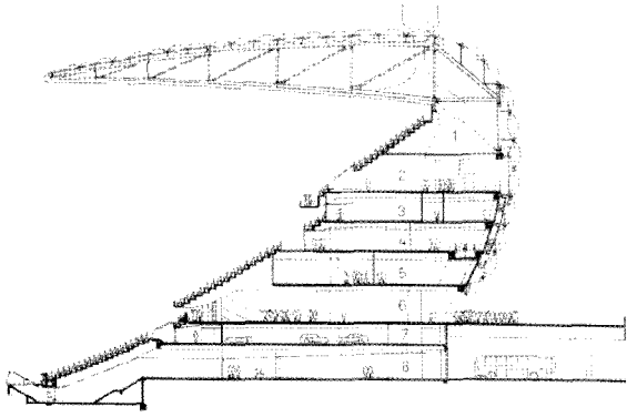
〈그림 6〉 알리안츠 아레나 단면
