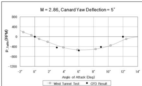
(d) Roll-rate of the freely spinning tailfins
