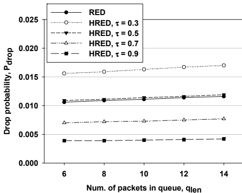
그림 5. HRED방식에서 히스토리 리스트 점유율 임계치 \tau 의 변화에 따른 drop확률의 변화
