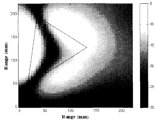
그림 10. 패치에 의한 수직 자계 분포 Fig. 10. The change of the Hz field by the sub patch.
