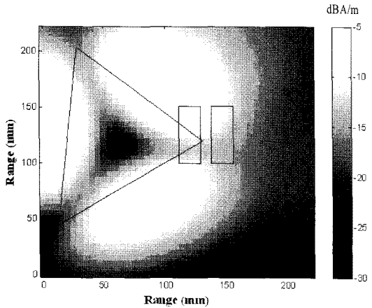
(a) 시뮬레이션 된 수직 자계 분포 (a) Simulated Hz field distribution
