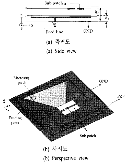
그림 2. 제안된 안테나 구조 Fig. 2. The structure of the proposed antenna.
