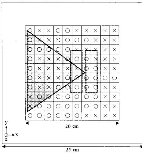
(b) 안테나 인식 영역 (b) Reading zone of the proposed antenna
