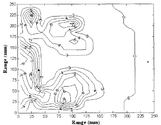
그림 4. 소형 근거리장 태그와의 인식거리 Fig. 4. The reading range using a small NF tag.
