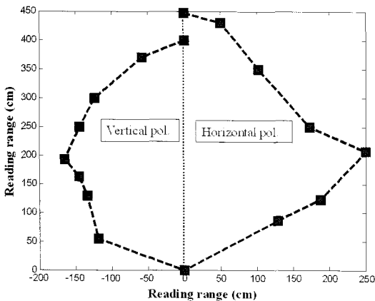
그림 9. 원거리장 인식 영역 Fig. 9. The reading range using a far-field tag.
