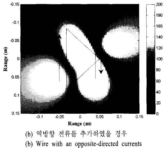
그림 1. 안테나 구조에 의한 수직 자계 분포 특성 Fig. 1. Characteristics of the H_z field distribution.
