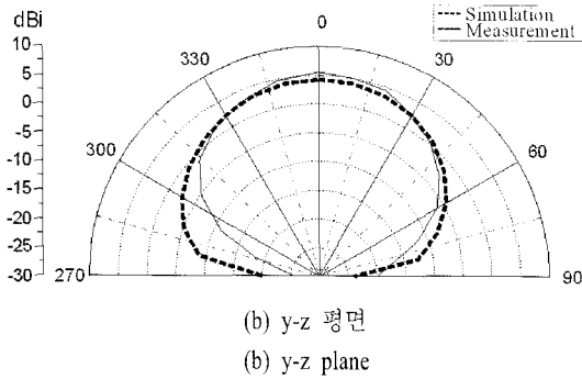
그림 8. 측정된 안테나 복사 패턴(912 MHz) Fig. 8. Measured radiation patterns of the antenna(912 MHz).
