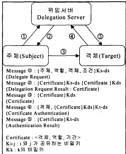
[그림 3] 일시적 권한 위임 프로토콜
