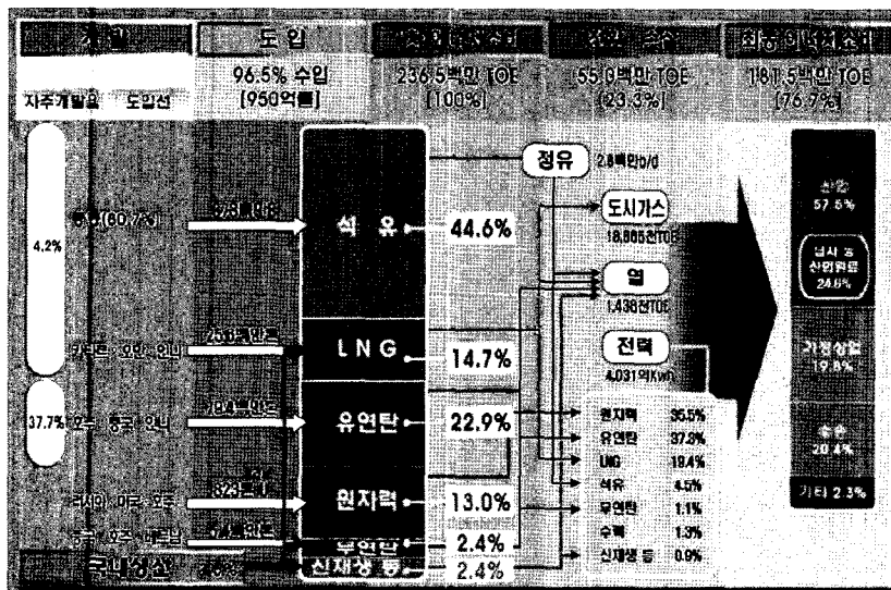
그림 1 우리나라 energy balance flow
