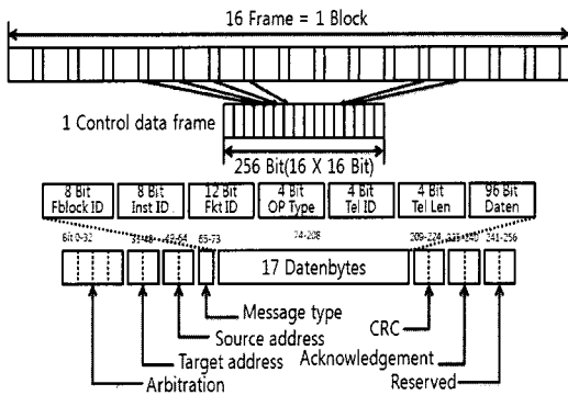
그림 3. MOST Control Channel Fig 3. MOST Control Channel
