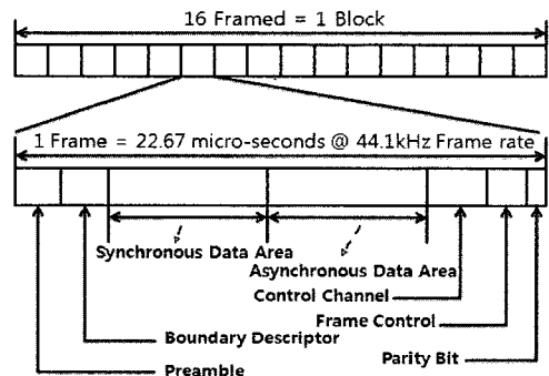
그림 2. MOST 전송 유형 Fig 2. MOST Transport Type
