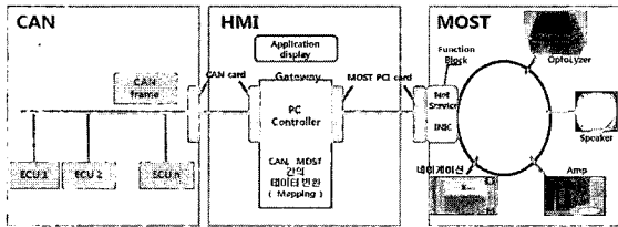
그림 5. 시스템의 구조도 Fig 5. Structure of System
