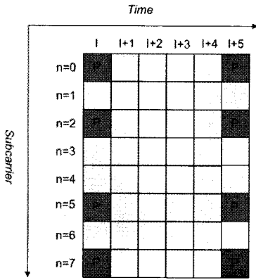
그림 2. TEDS 데이터 버스트 구조
