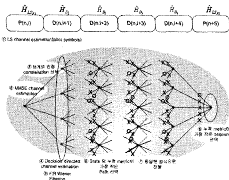
그림 6. 제안된 채널 추정 과정
