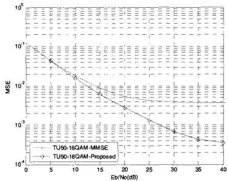
(a) TU50 채널에서 MSE
