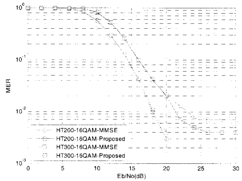
그림 9. 16-QAM, HT200 채널에서의 추정 오류의 영향
