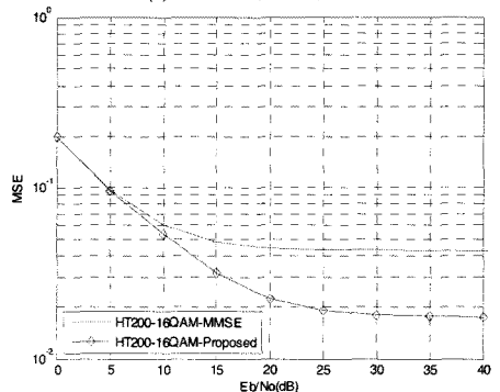
(b) HT200 채널에서 MSE
