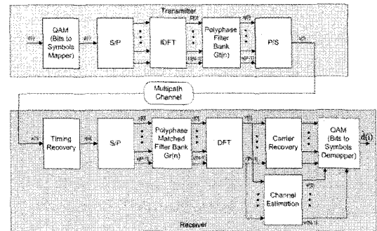
그림 1. FBMCM 송수신기 구조
