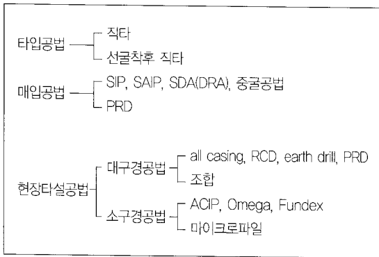
그림 1. 시공법에 따른 말뚝공법의 분류
