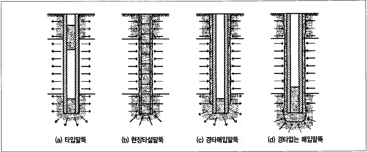
그림 2. 말뚝 설치 시 주변 흙의 이동
