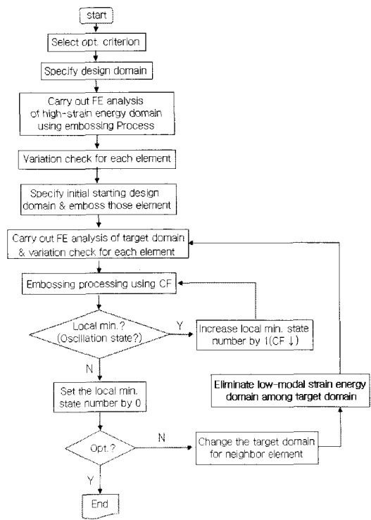
[그림 1] 순서도
