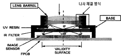
[그림 1] 초소형 barrel, base 조립 구조
