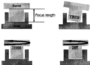
[그림 3] 플라스틱 barrel, base의 조립토크 불량 유형
