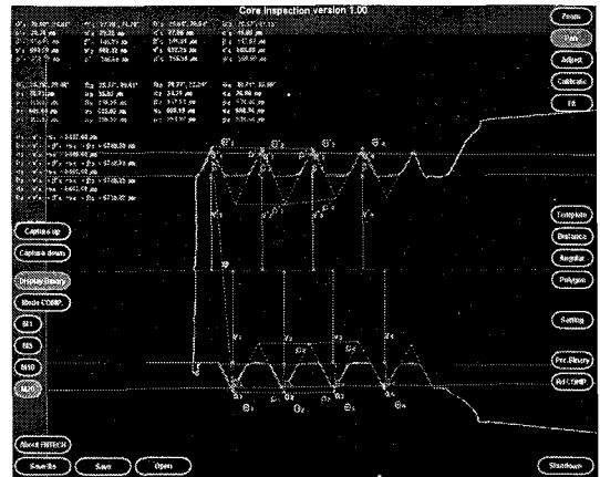
[그림 12] 이진화 및 경계 검출 과정을 통한 나사코어 주요 기하 측정
