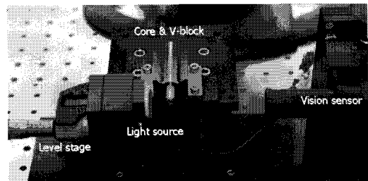
(b) 측정부 세부 모듈
