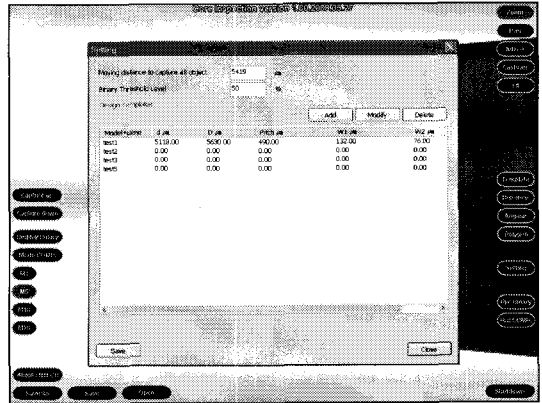
[그림 11] 코어 및 전극의 주요 설계 형상 기하 입력창
