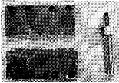
[그림 5] 나사형상 전극과 슬라이드 코어(barrel 성형용)
