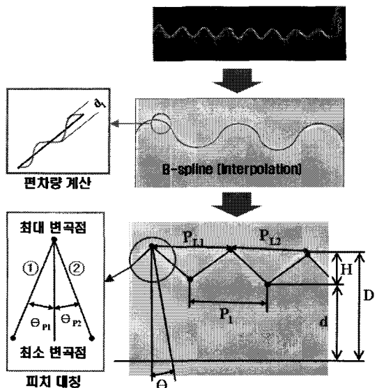
[그림 7] 사출 성형품 측정 파라미터 선정
