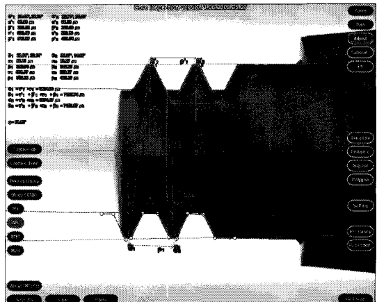
[그림 13] 측정 이미지상 나사코어 주요 기하 측정
