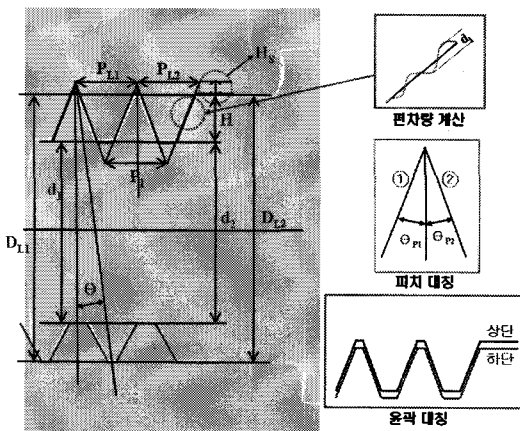
[그림 6] 나사코어 및 전극 측정 파라미터 선정
