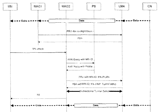
그림 2. PMIPv6에서 MN의 핸드오프 절차
