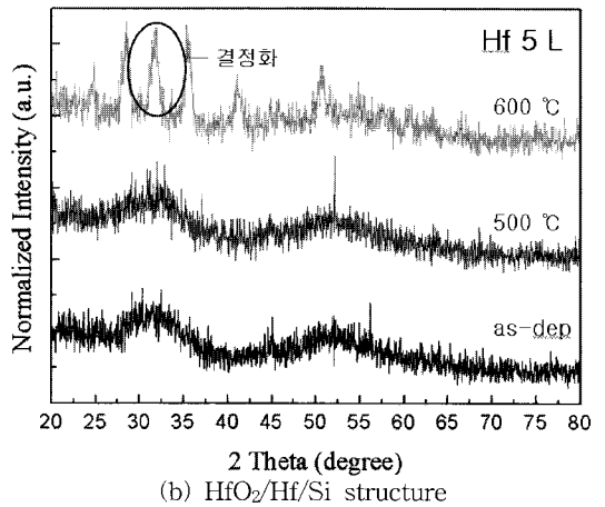
그림 3. 열처리 온도에 따른 (a) HfO 2 박막 및 (b) HfO 2 /Hf 박막의 XRD 스펙트라. Fig. 3. XRD spectra of a deposited (a) HfO 2 and (b) HfO 2 /Hf films.
