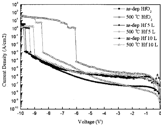
그림 4. Hf metal layer 두께에 따른 HfO 2 MOS capacitor의 I-V 특성.
