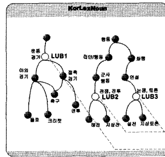
그림 5 KorLexNoun과 KorLexVerb 간 논항의 선택 제약 연동2
