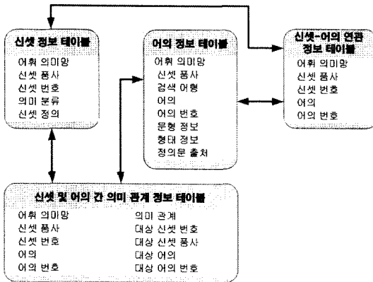
그림 6 KorLex 의미정보 구조
