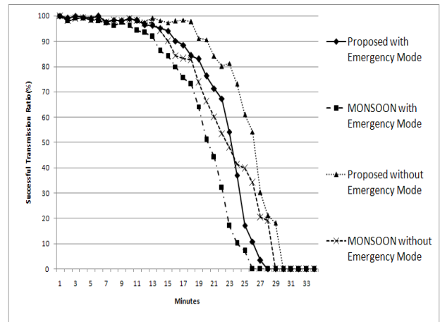
(그림 9) 시간에 따른 Class 2 데이터 전송 성공률
