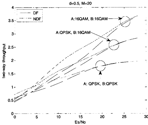
그림 4. SNR에 따른 양방향 협력 ARQ 프로토콜의 성능비교
