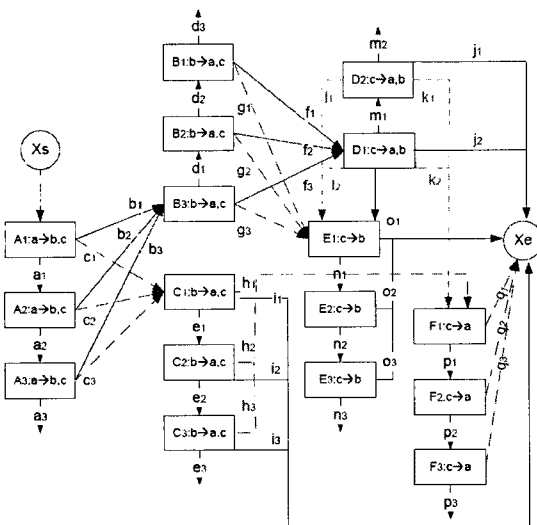
그림 2. 양방향 협력통신 프로토콜의 스테이트 다이어그램
