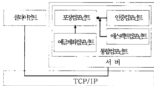
그림 8. 컴포넌트의 보안모델을 사용한 응용시스템의 구조 Fig 8. The Application Architecture for Security Model of Component
