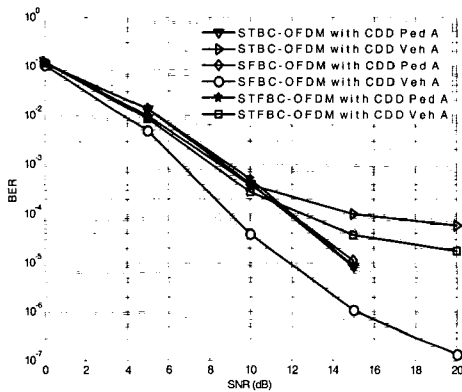
Fig. 8. STBC/SFBC/STFC-OFDM w. CDD
