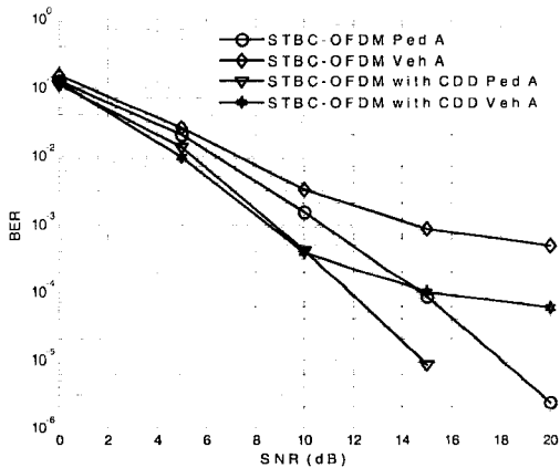
Fig. 5. STBC-OFDM vs. STBC-OFDM w. CDD
