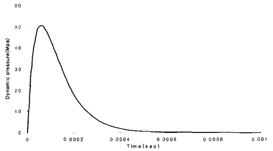
그림 5. 발파하중
