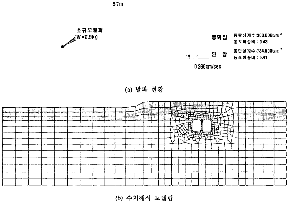
그림 7. 발파현황 및 수치해석 모델
