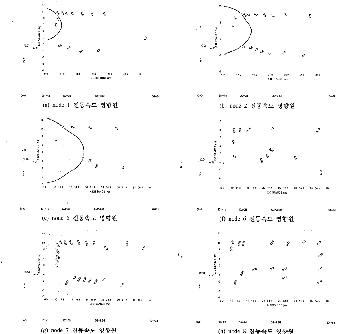
그림 12. 터널 라이닝 위치별 진동 영향원
