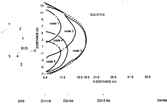
그림 13. 허용진동속도의 대표포락선
