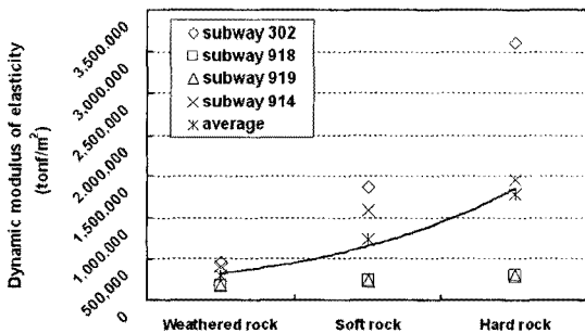
(a) 동탄성계수
