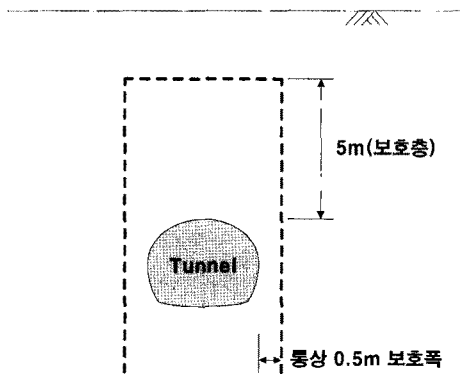
그림 3. 일본의 통상적 터널 보호영역
