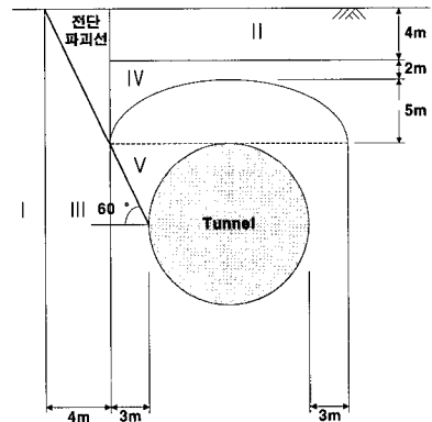
그림 2. 부산지하철 1호선 건설 시 터널 안전영역(1호선 기준)
