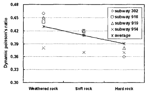
(b) 동포아송비
