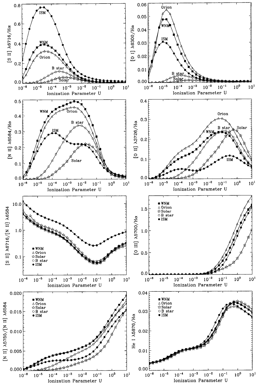
그림 3.— 평면 평행을 가정했을 때 이온화 인수 U 에 따른 방출선의 비, [S II] \lambda 6716/H\alpha , [N II] \lambda 6583/H\alpha , [O I] \lambda 6300/H\alpha , [O II] \lambda 3726/H\alpha , [O III] \lambda 5700/H\alpha , He I \lambda 5876/H\alpha , [S II] \lambda 6716/[N II] \lambda 6583 , [N II] \lambda 5755/[N II] \lambda 6583 의 변화
