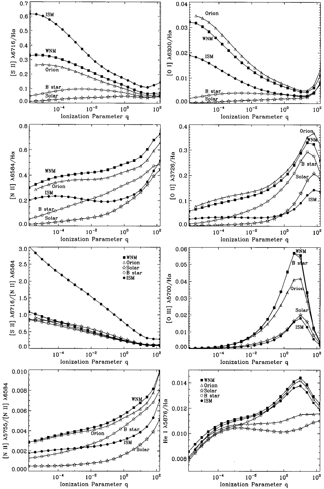
그림 2.— 구대칭을 가정했을 때 이온화 인수 q 에 따른 방출선의 비, [S II] \lambda 6716/H\alpha , [N II] \lambda 6583/H\alpha , [O I] \lambda 6300/H\alpha , [O II] \lambda 3726/H\alpha , [O III] \lambda 5700/H\alpha , He I \lambda 5876/H\alpha , [S II] \lambda 6716/[N II] \lambda 6583 , [N II] \lambda 5755/[N II] \lambda 6583 의 변화.
