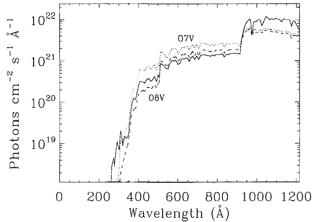
그림 1.— Hipparcos 항성 목록 (Perryman et al. 1997)의 OB형 별들의 항성 스펙트럼을 평균하여 구해진 스펙트럼. 비교를 위해 O7V 및 O8V형의 항성 스펙트럼을 함께 나타내었다.
