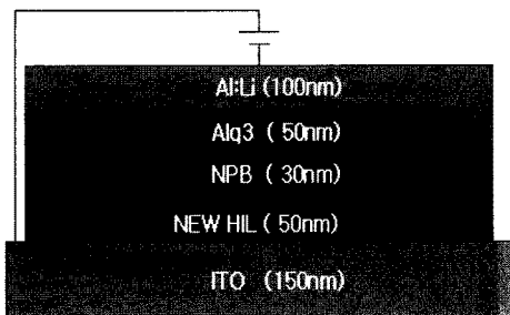
그림 1. 제작한 OLED 소자의 구조.
