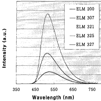
그림 6. 정공주입재료에 따른 OLED 소자의 발광 스펙트럼.
