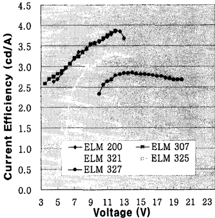
그림 4. 정공주입재료에 따른 OLED 소자의 인가 전압에 대한 발광전류효율.
