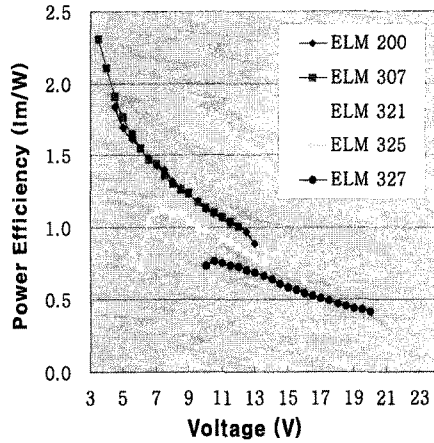
그림 5. 정공주입재료에 따른 OLED 소자의 인가 전압에 대한 발광전력효율.
