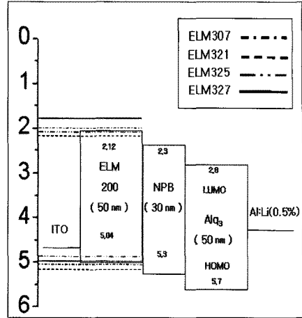
그림 7. 정공주입재료에 따른 OLED 소자의 에너지 준위.
