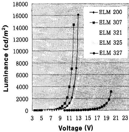
그림 3. 정공주입재료에 따른 OLED 소자의 인가 전압에 대한 발광휘도.
