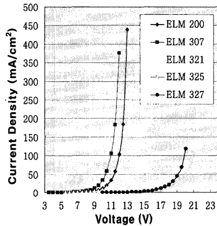
그림 2. 정공주입재료에 따른 OLED 소자의 인가전압에 대한 전류밀도.
