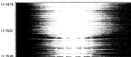
그림 7. 전파품질측정 스펙트로그램 결과
