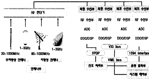
그림 2. 차세대 지능형 전파감시 시스템 구성도
