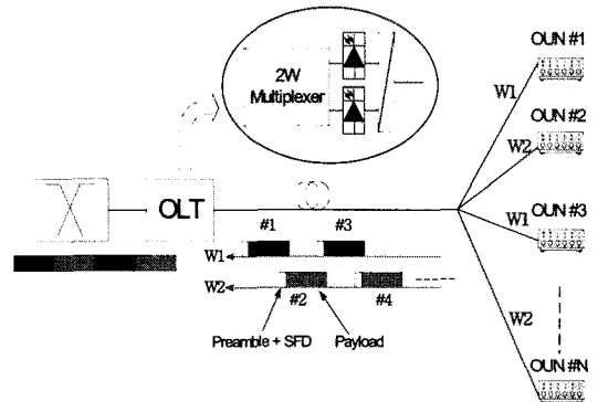
그림 2. 2W-PON 시스템의 구조
