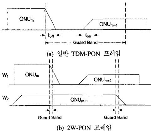
그림 1. 일반 TDM-PON과 제안된 2W-PON 가드밴드 비교
