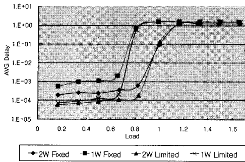
그림 5. GE-PON과 제한된 2W-PON 전송지연 비교
