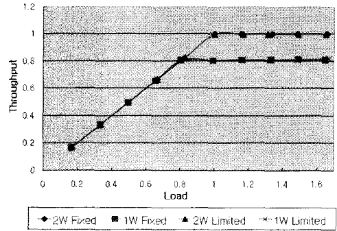
그림 4. GE-PON과 제안된 2W-PON 전송효율 비교
