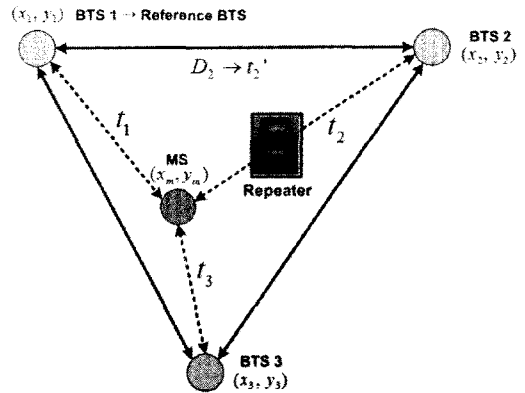
그림 3. 제안하는 중계기 보정 알고리즘
