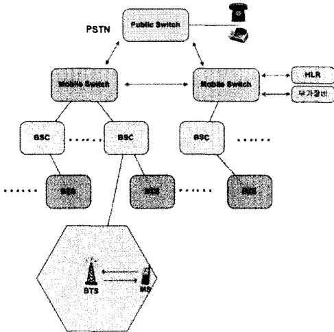
그림 1. CDMA 시스템 구성도
