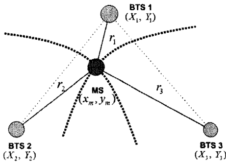
그림 6. TDOA 알고리즘을 이용한 위치 측위
