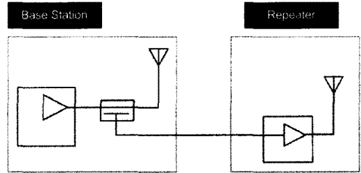
그림 2. 중계기 구조
