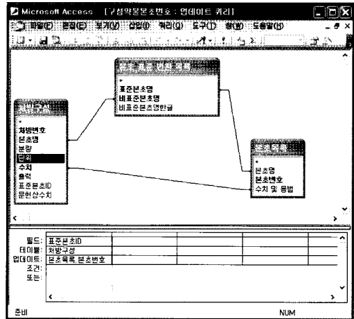
그림 7. 구성본초 본초번호 업데이트 쿼리
