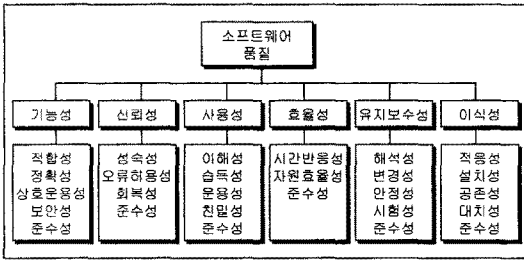
그림 3. ISO/IEC 9126 소프트웨어 제품품질 Fig. 3. Product Quality of Software ISO/IEC 9126
