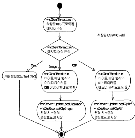
그림 7. 개발된 VNC 서버가 클립보드 콘텐츠를 원격시스템의 클립보드에 저장하는 과정 Fig. 7 Procedure for the developed VNC server to store the received clipboard content
