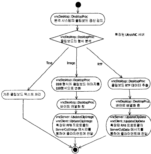
그림 3. 개발된 VNC 서버가 원격시스템의 클립보드 콘텐츠를 클라이언트로 전송하는 과정 Fig. 3. Procedure for the developed VNC to send the clipboard content of the remote system to clients
