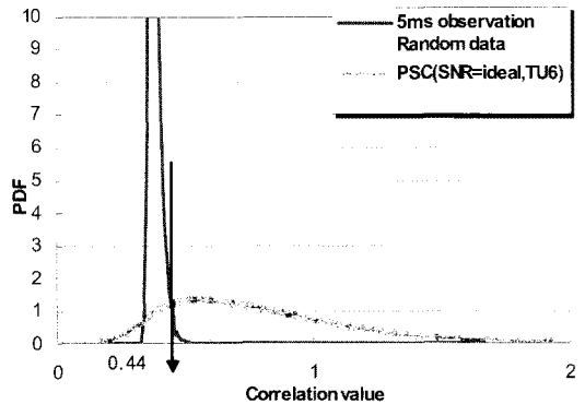
그림 14. 상관 출력의 PDF 분석
