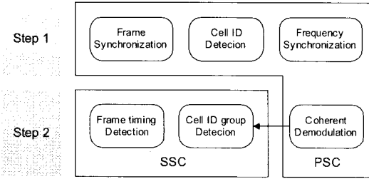
그림 4. 초기 셀 탐색 모식도
