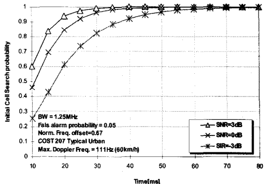
그림 18. 셀 탐색 시간에 따른 초기 셀 탐색 성공 확률
