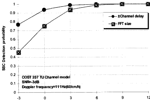
그림 16. SNR에 따른 SSC 검출 확률 비교
