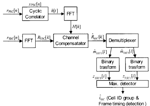
그림 10. SSC 검출 수신기 구조
