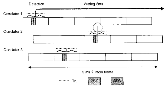
그림 9. PSC 검출기의 대기 상태
