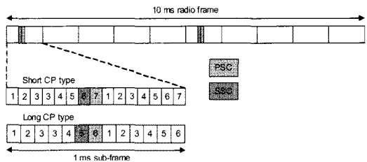
그림 1. Downlink FDD 모드의 프레임 구조 예시도
