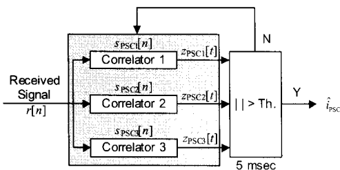
그림 8. 다중 셀을 고려한 PSC 검출 수신기 구조
