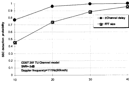
그림 17. 셀 탐색 시간에 따른 SSC 검출 확률 비교
