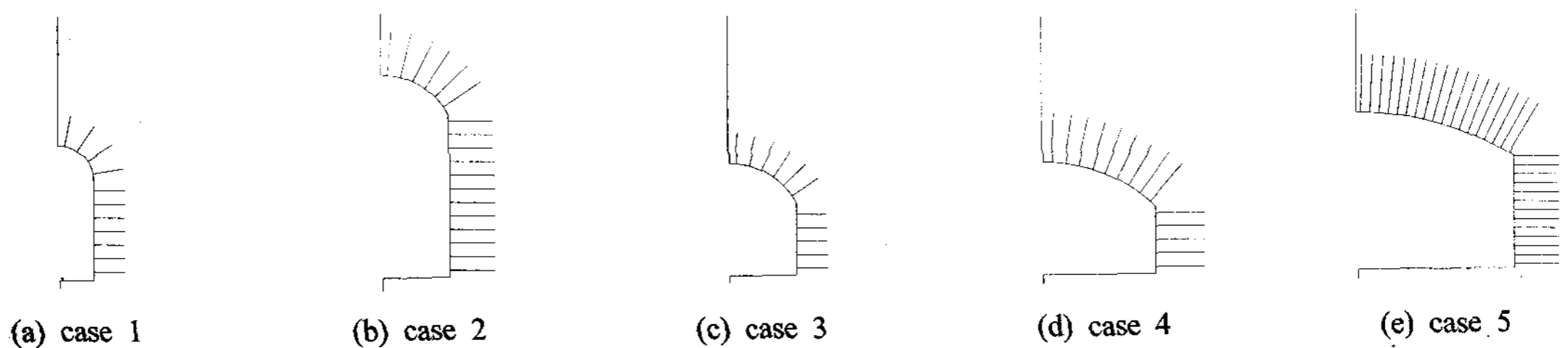
그림 3. case별 rockbolt 보강패턴
