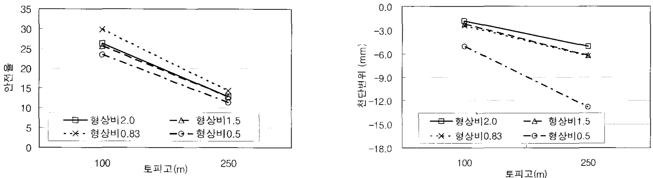
(a) 토피고에 대한 안전율의 영향
