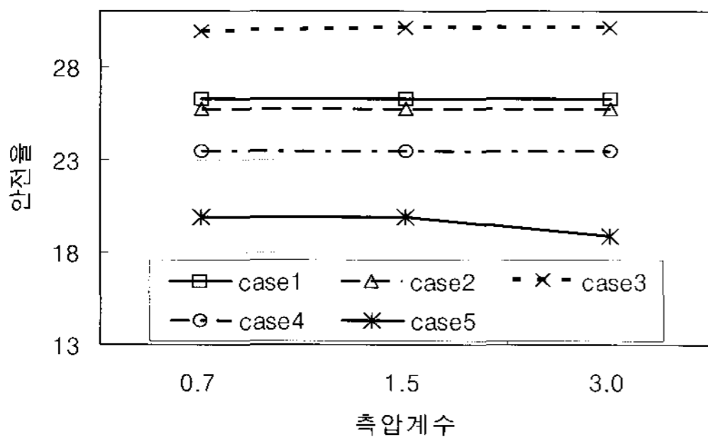
(a) 측압계수와 안전율의 관계
