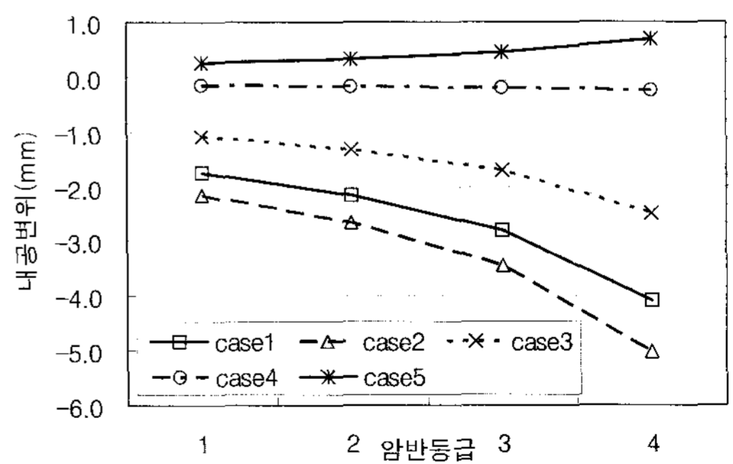
(b) 암반등급에 대한 측벽부 내공변위
