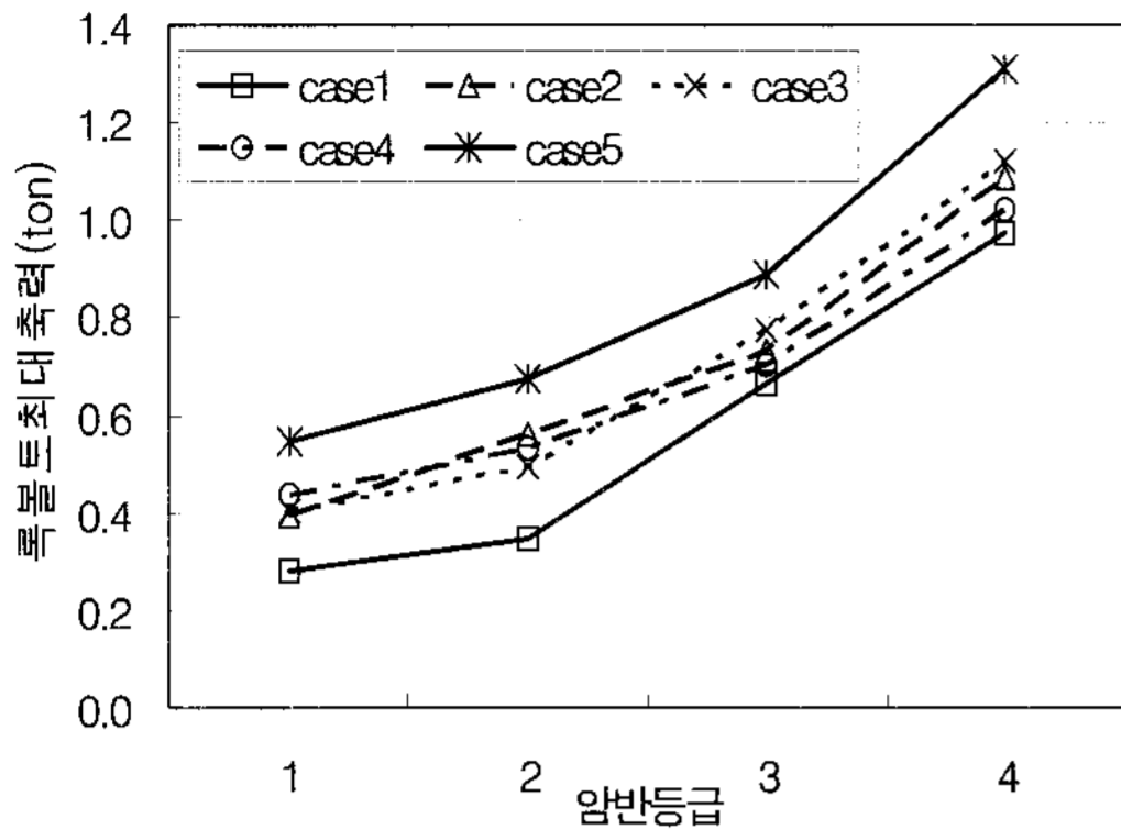
(a) 토피고 100 m
