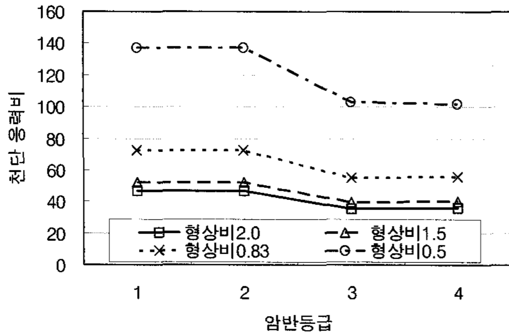
(a) 천단부 응력비
