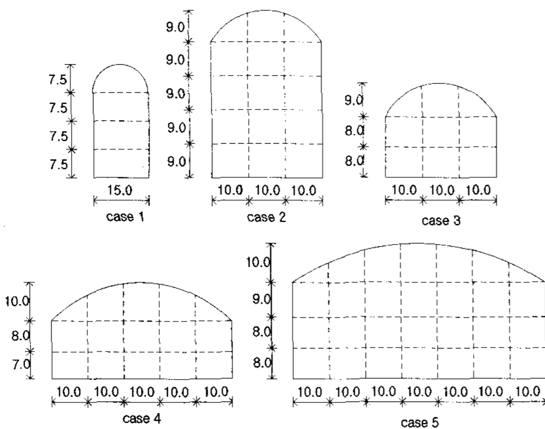
그림 1. 가정된 지하공동 형상
