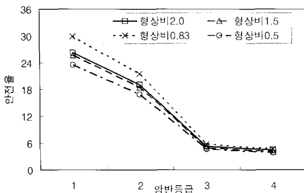
(a) 토피고 100 m
