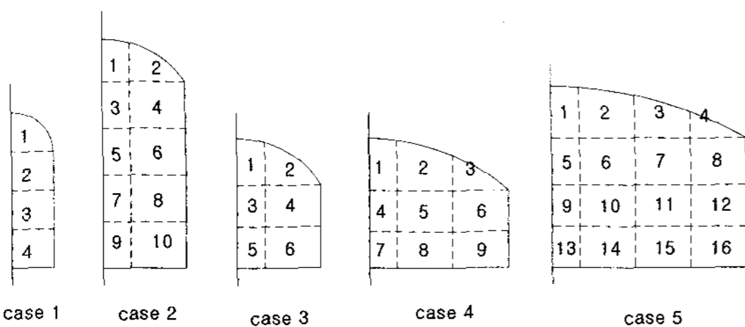
그림 2. 수치해석 지하공동형상과 지하공동 굴착순서
