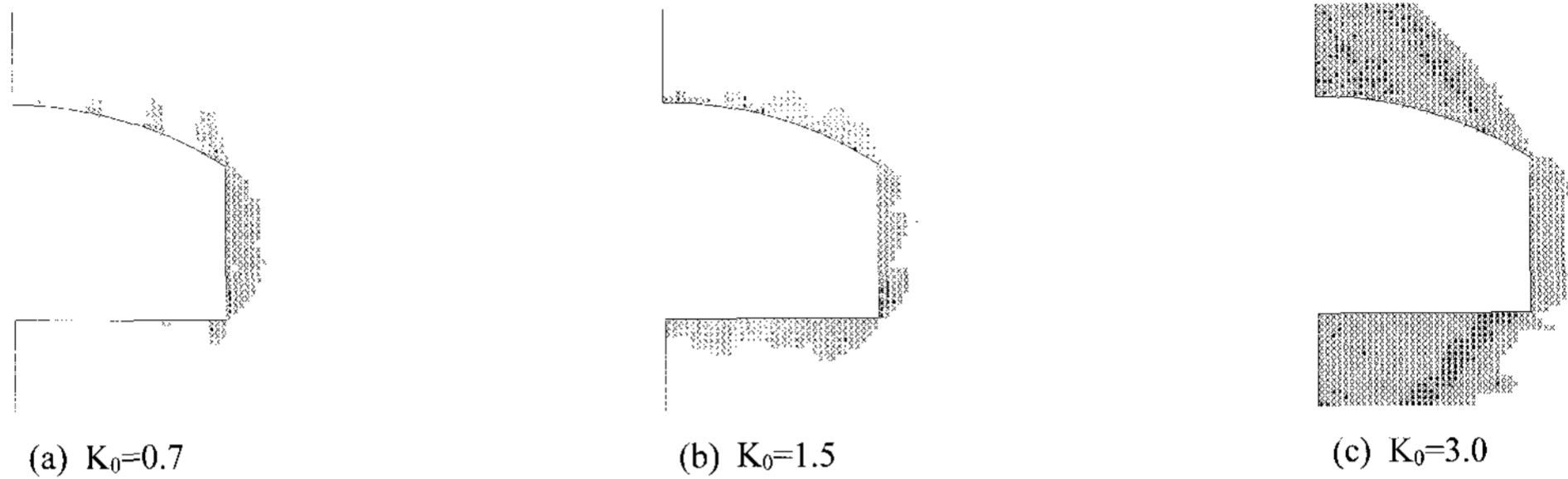
그림 4. 측압계수에 대한 소성영역(case 5, 암반 4등급, 토피고 250 m)
