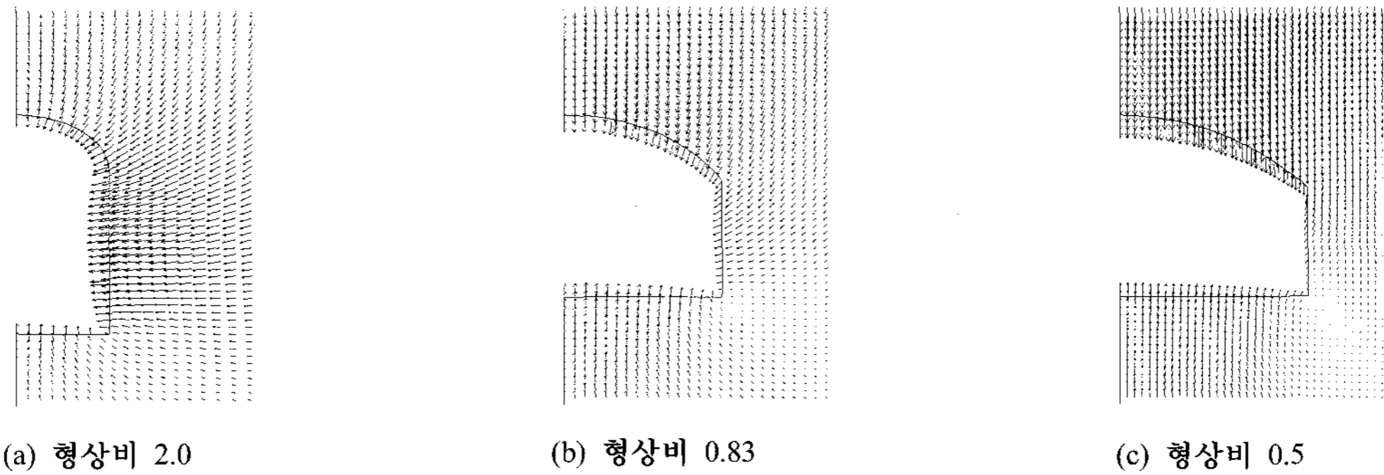
그림 7. 형상비에 대한 변위벡터도(암반 4등급, 측압 0.7)
