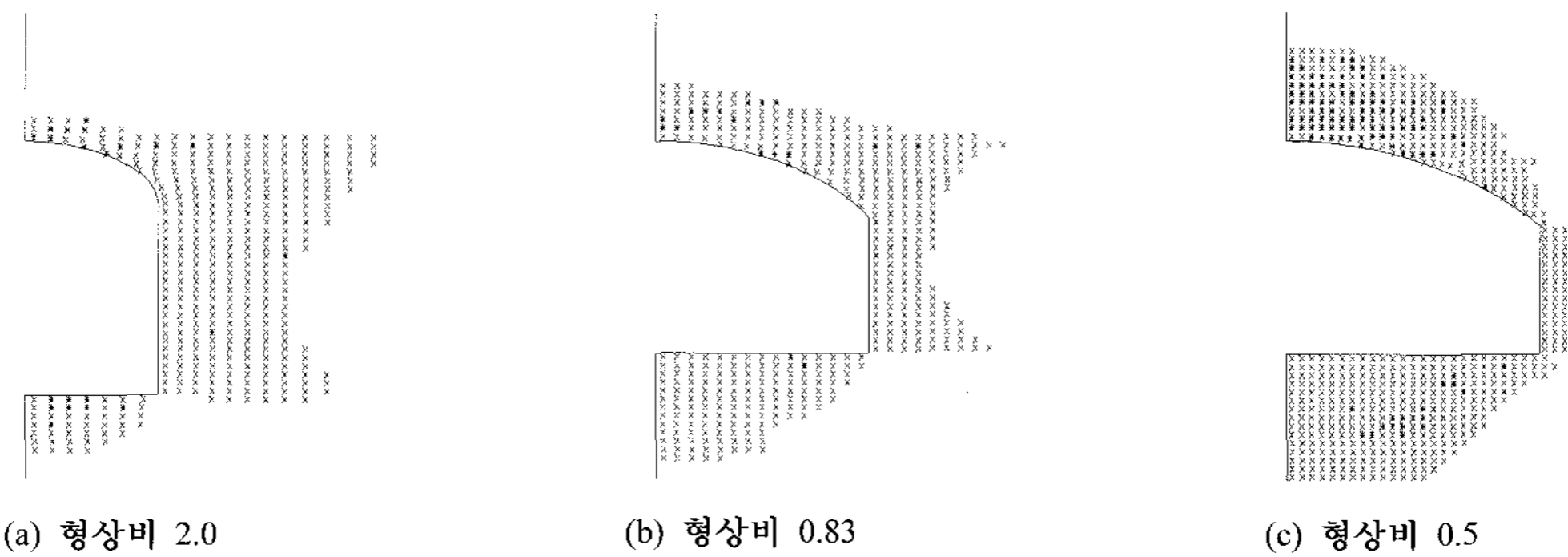
그림 8. 형상비에 대한 소성영역(암반 4등급, 토피 250 m, 측압 3.0)
