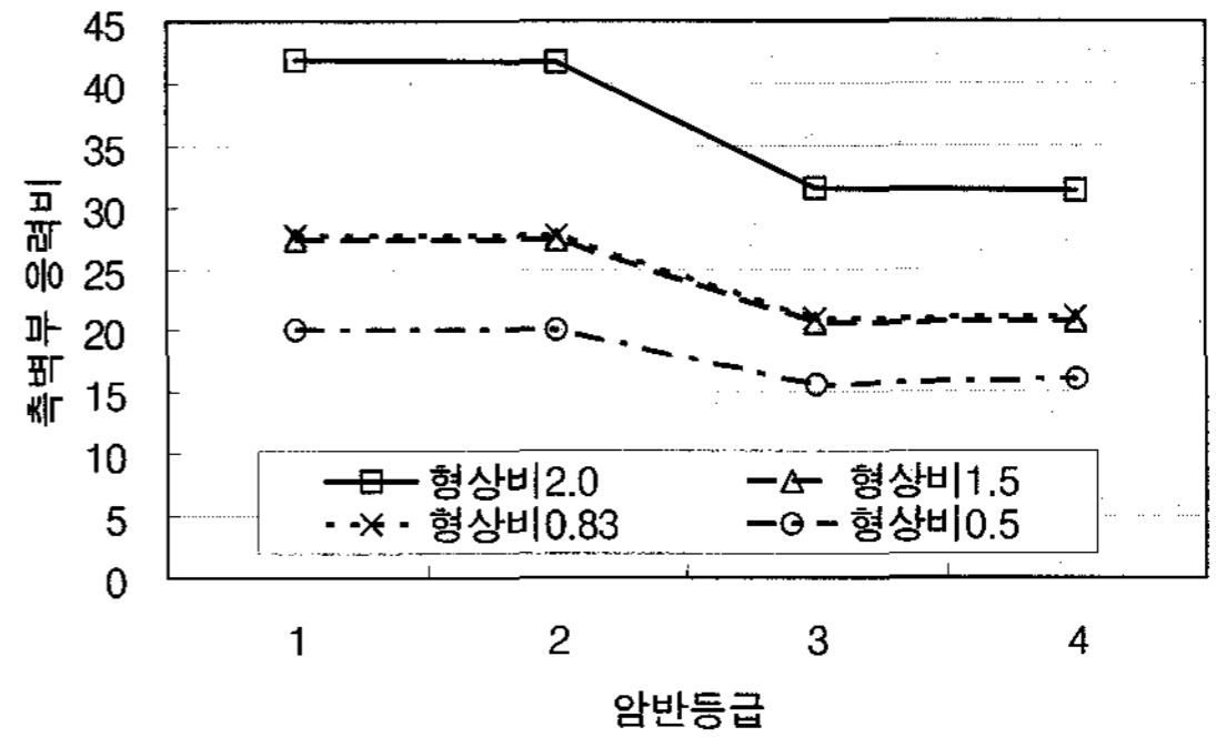
(b) 측벽부 응력비
