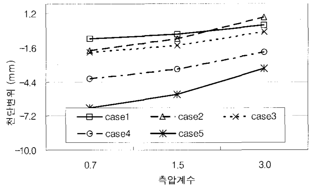
(b) 측압계수와 천단변위의 관계
