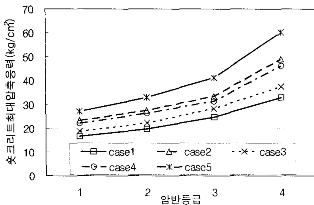
(a) 암반등급에 대한 숏크리트최대압축응력
