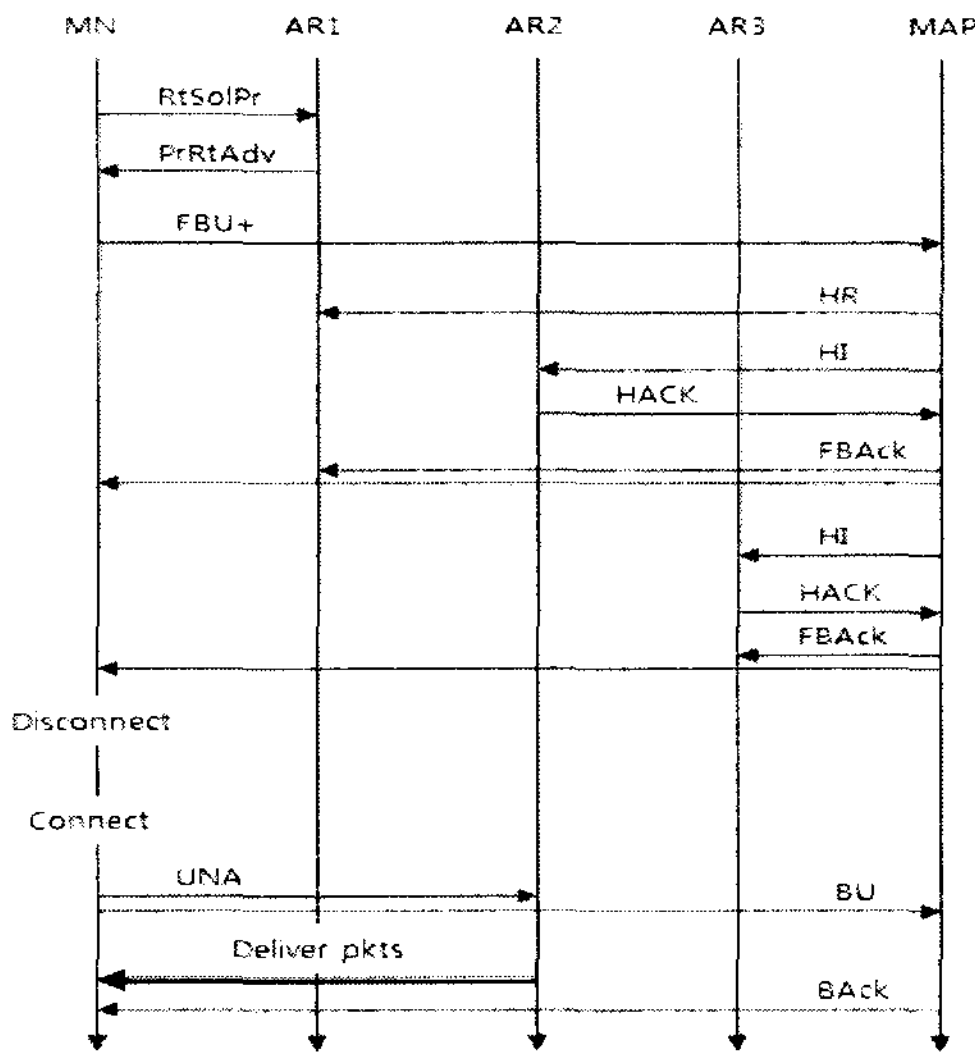
그림 1. 개선된 HIMIPv6의 Intra-MAP 핸드오버
