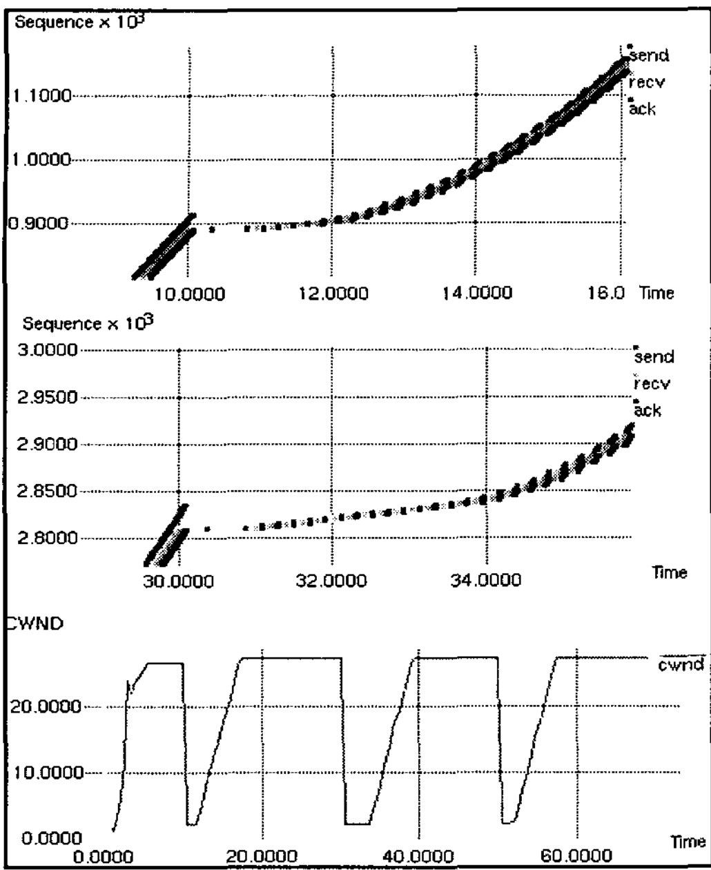
그림 7. TCP Vegas에서 HMIPv6동작
