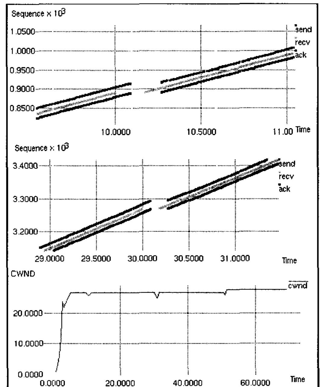
그림 9. TCP Vegas에서 HIMIPv6동작
