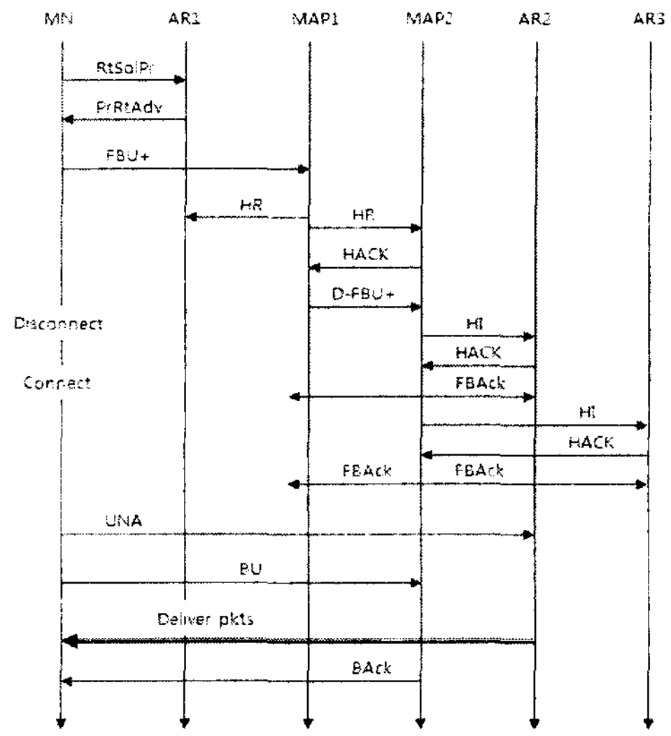
그림 2. 개선된 HIMIPv6의 Inter-MAP 핸드오버
