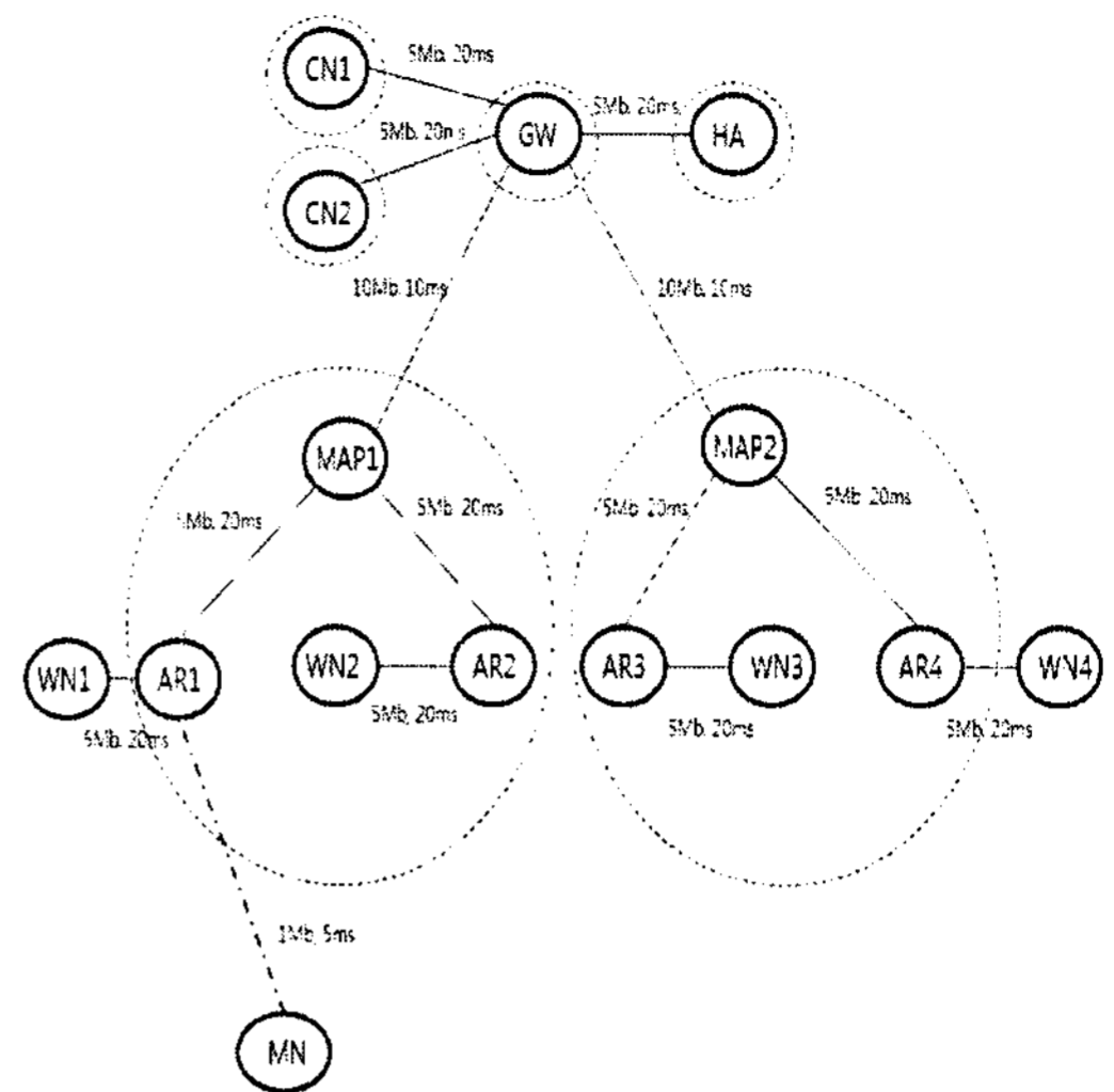
그림 3. 실험 토폴로지
