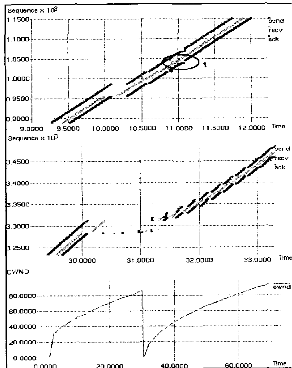
그림 5. TCP Tahoe에서 FMIPv6 동작
