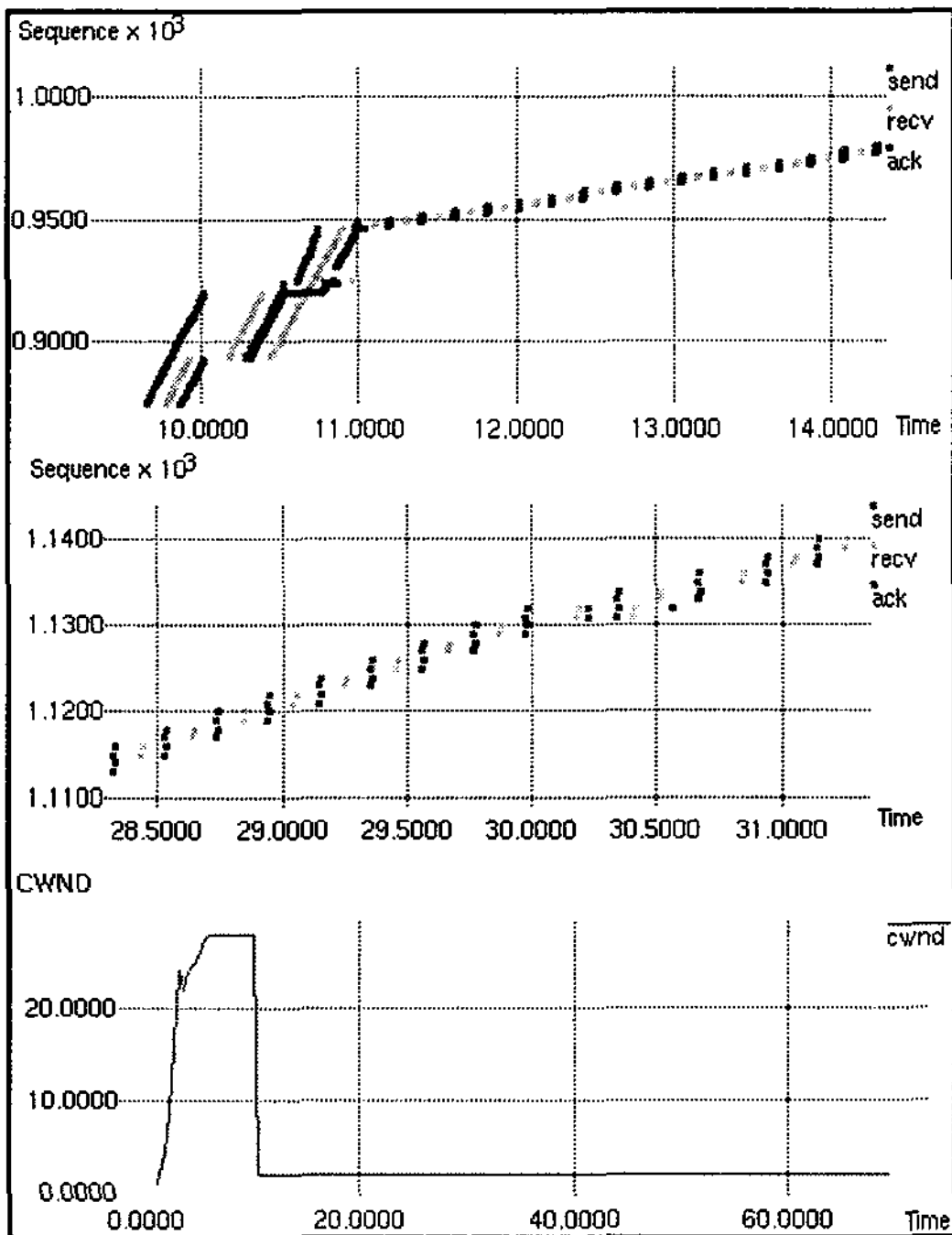
그림 8. TCP Vegas에서 FMIPv6동작
