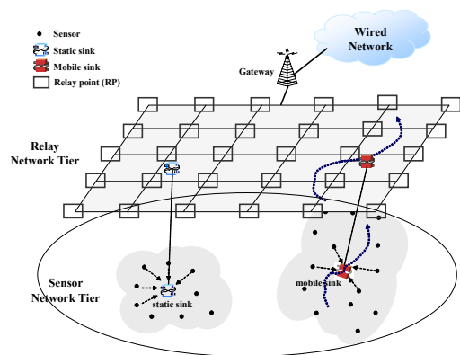
(그림 2) 3-계층 무선 센서 망 구조
