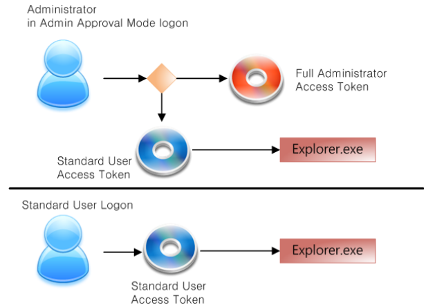
(그림 6) Windows Vista UAC 동작 메커니즘
