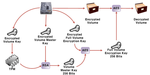
(그림 2) TPM만을 사용하여 BitLocker를 적용한 경우
