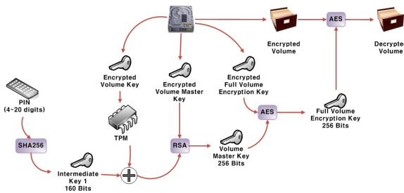
(그림 3) TPM과 PIN을 사용하는 BitLocker를 적용한 경우
