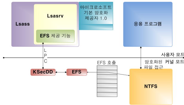
(그림 9) EFS 구조
