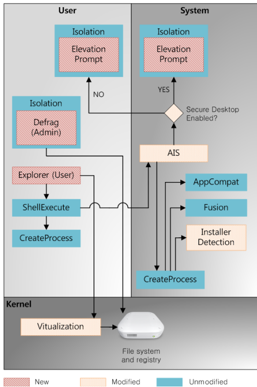
(그림 7) Windows Vista UAC구조
