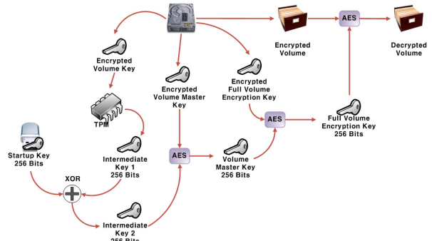
(그림 4) TPM과 USB dongle(Startup-key)를 사용하여 BitLocker를 적용한 경우
