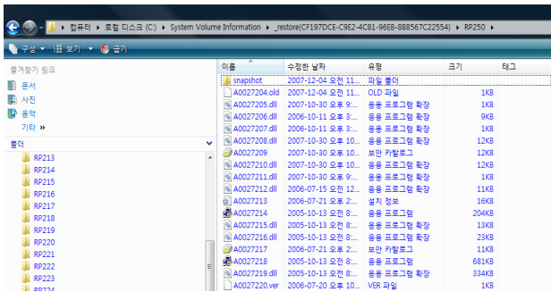
(그림 12) Shadow copy & Volume Snapshot 저장
