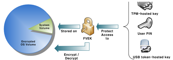
(그림 1) BitLocker 보안 메커니즘
