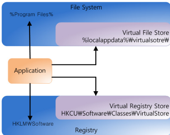
(그림 8) UAC의 가상화
