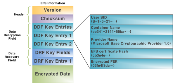
(그림 10) EFS 정보의 구조와 키 엔트리
