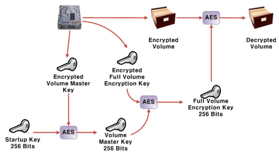
(그림 5) TPM 없이 BitLocker를 적용한 경우
