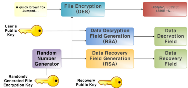
(그림 11) EFS 암호화 메커니즘
