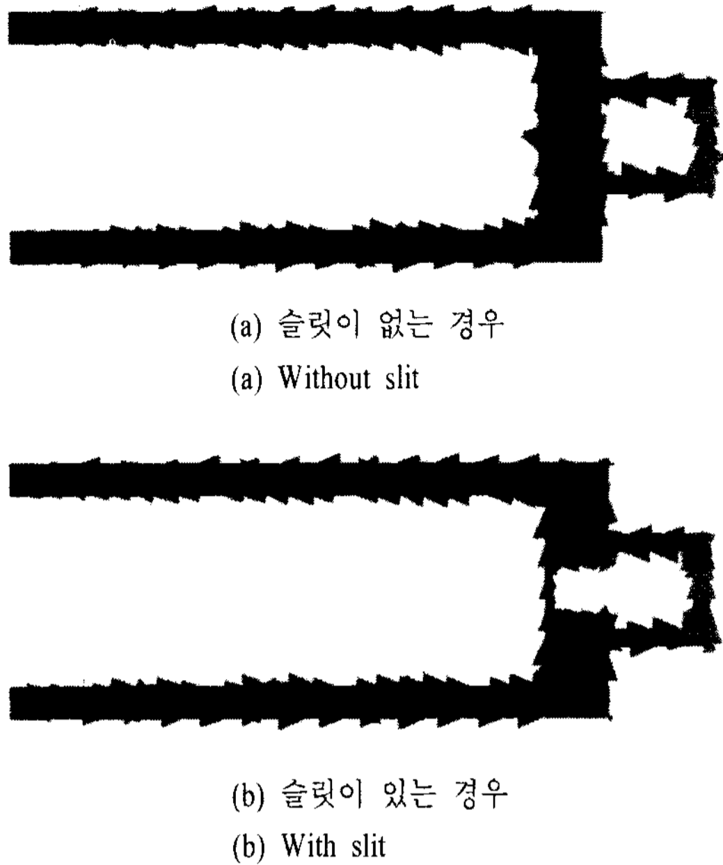
그림 10. 최적화된 태그 안테나의 표면 전류 분포 Fig. 10. Current distribution of the optimized tag antenna.
