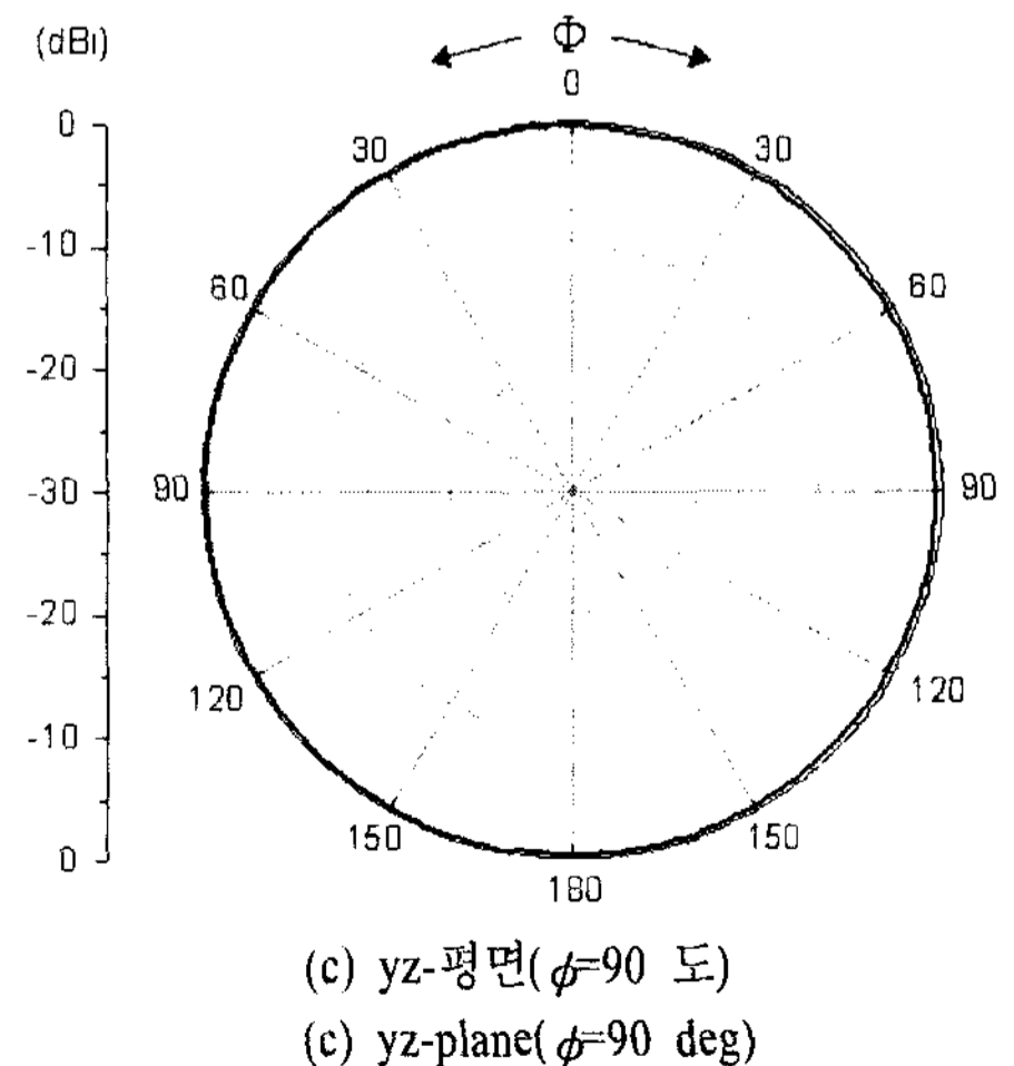
그림 11. 최적화된 태그 안테나의 복사 패턴 Fig. 11. The radiation pattern of the optimized tag antenna.
