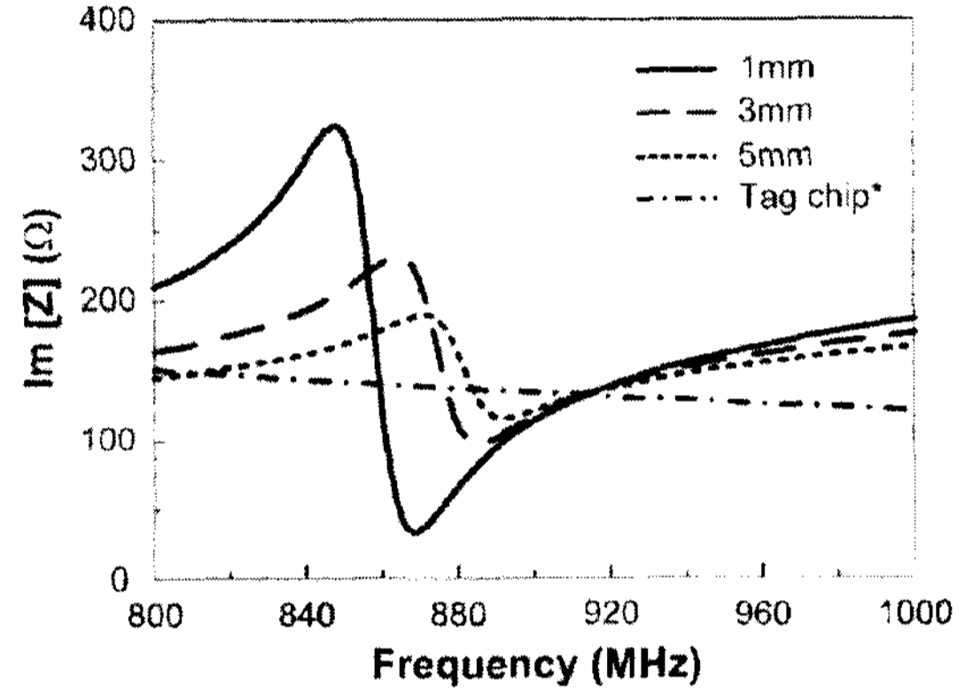
(b) 입력 리액턴스 (b) Input reactance
