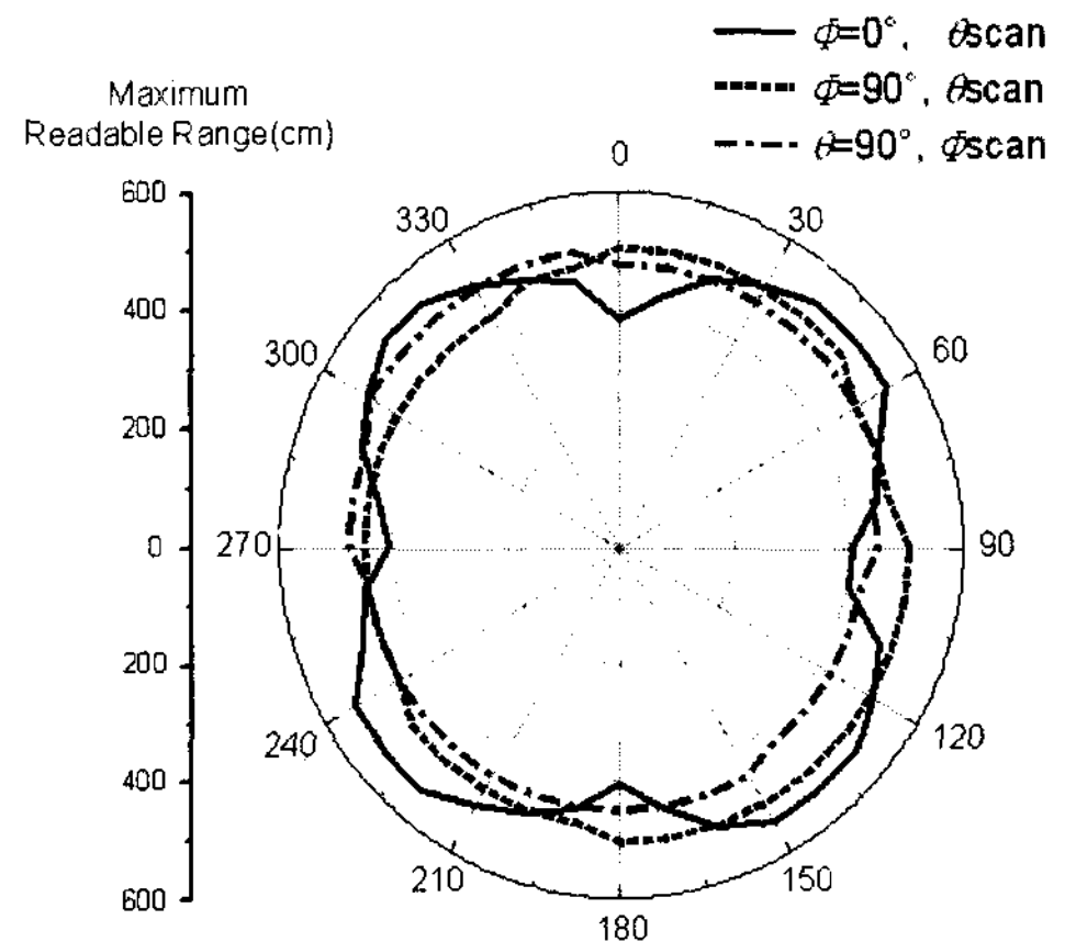
그림 13. 최적화된 슬릿이 없는 태그 안테나의 인식 거리 특성
