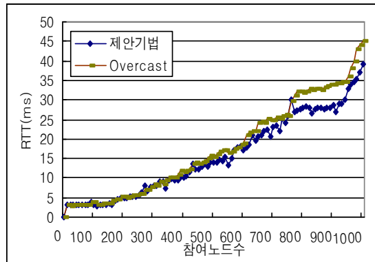
그림 8 참여노드 수에 따른 RTT 측정 Fig. 8 RTT for the join node number of times
