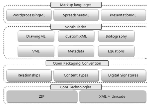
그림 4. OOXML의 주요 구조 Fig 4. The Essential Scheme of the OOXML
