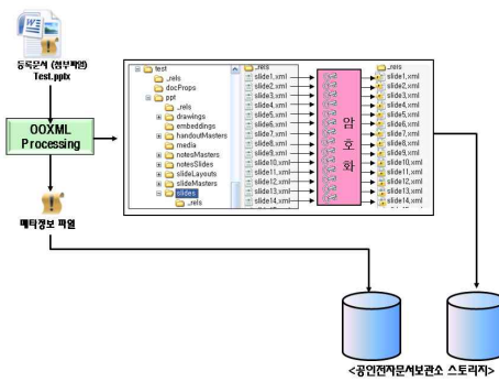
그림 7. OOXML 기반의 처리 절차 Fig 7. operation process on the based COOXML
