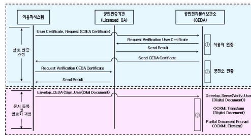
그림 6. 상호인증 절차와 문서 등록 및 암호화 과정 Fig 6. Mutuality Certification procedures and Document Registration and cryptograph process
