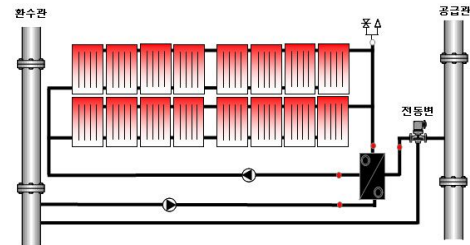
그림 3. 지역난방수 축열조 가열 정온방식
