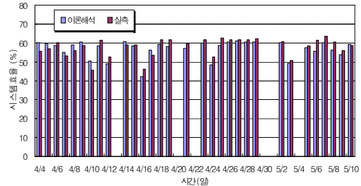
그림 13. 진공관형 집열부의 집열효율
