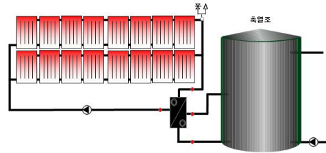
그림 2. 보충수 예열방식
