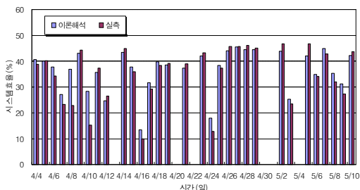
그림 12. 평판형 집열부의 집열효율
