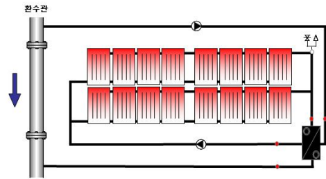
그림 1. 지역난방수 환수 승온방식
