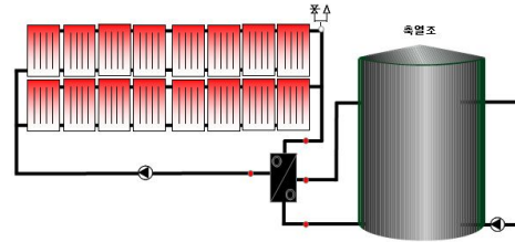
그림 3. 지역난방수 축열조 가열 정온방식
