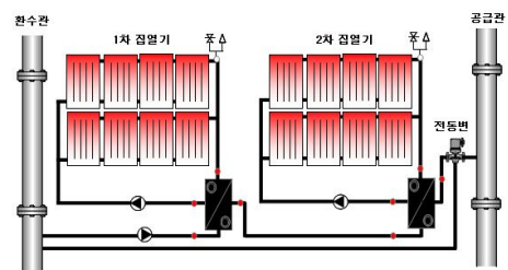
그림 5. 정온 공급방식(복합 집열부형)
